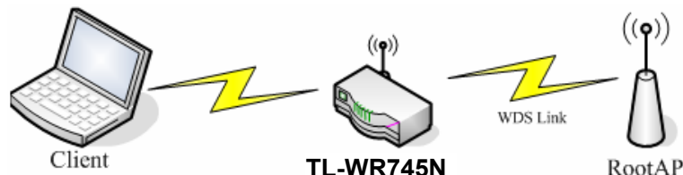
图 5-11 WDS 连接拓扑图
