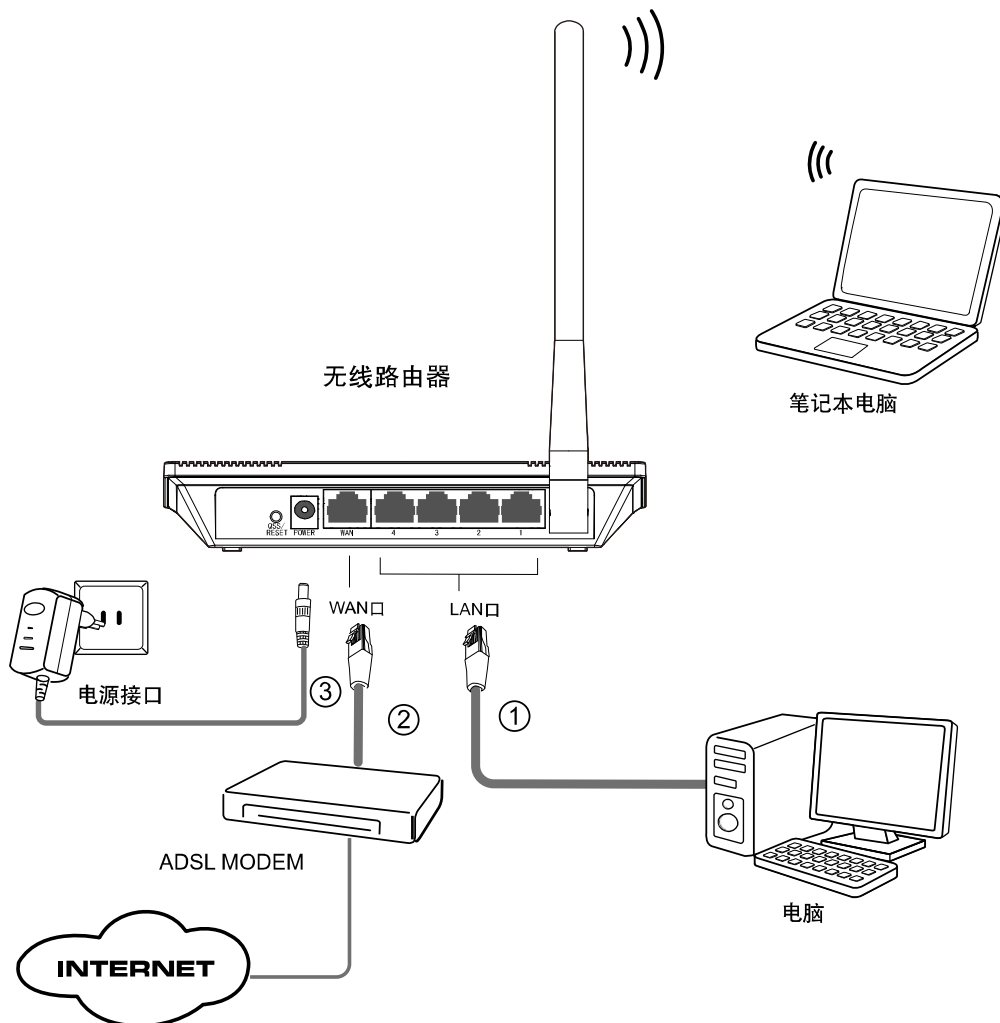
图 4-1 TL-WR745N 硬件安装示意图
