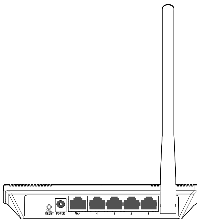
图 3-2 TL-WR745N 后面板示意图
